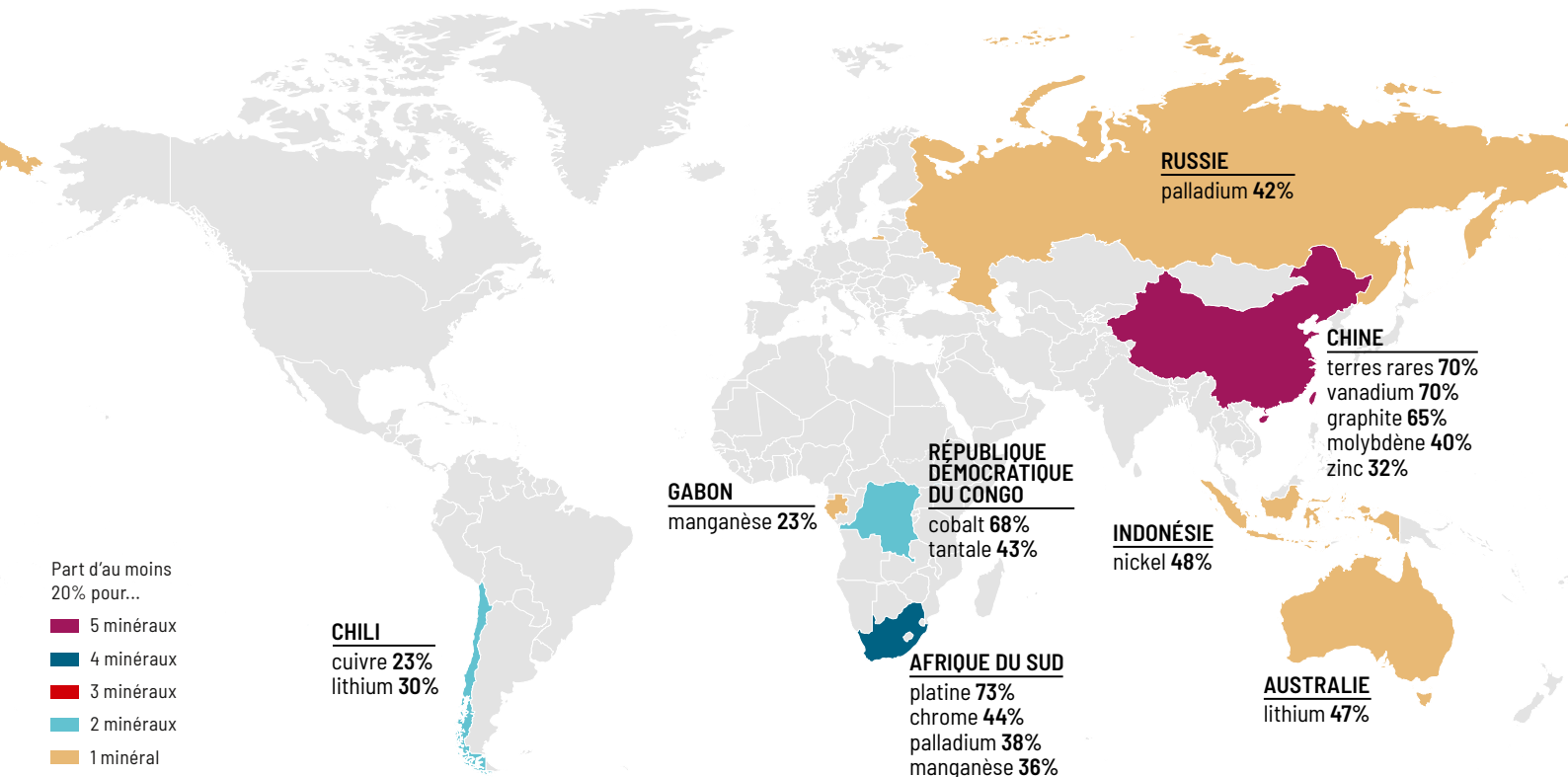
Figure 5: Concentration géographique de l'extraction de minéraux essentiels pour la transition énergétique (source: U.S. Geological Survey).
